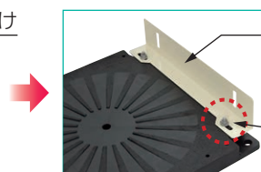
②ベース取り付け
